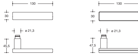
Modell 185X
