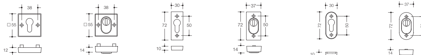
Schutzrosette 308X..ES...
