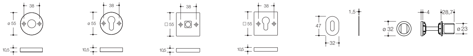
Drückerrosette 305...X..
