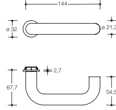
Modell 111XAM
