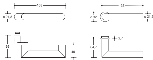
Modell 162XAM
